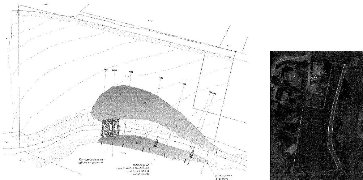
Figure 2 : vue en plan et localisation parcellaire du piège à graviers
