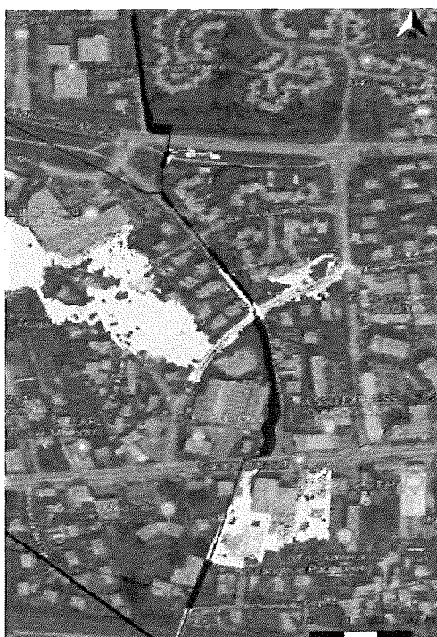
Figure 7 : carte des zones inondables en état de projet pour une Q10 (secteur aval de Bourgoin-Jallieu)
