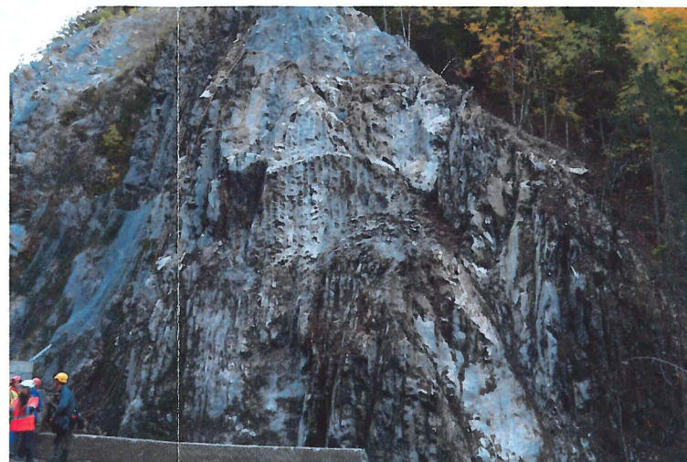
Terrassements rocheux à la future tête aval du tunnel des Cliets
