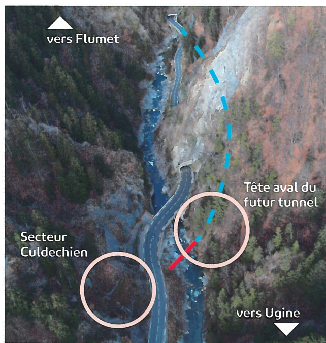
Plan de situation des zones de travaux
