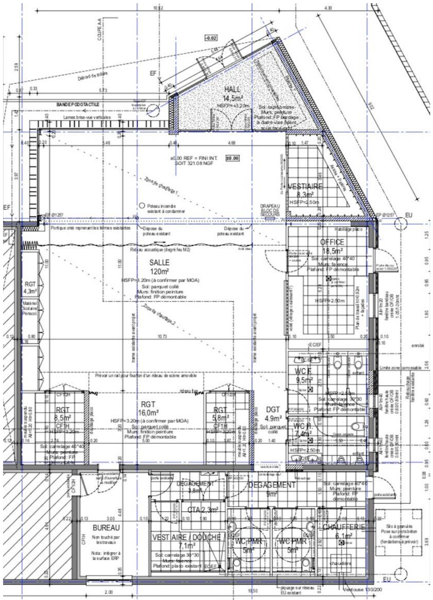
Plan de la Salle Kauffmann & Wassmer Architectes
